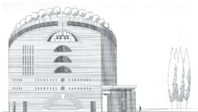
Cathédrale d'Évry, plan, élévation nord, 1989. Architecte : Mario Botta. — 781W/52
